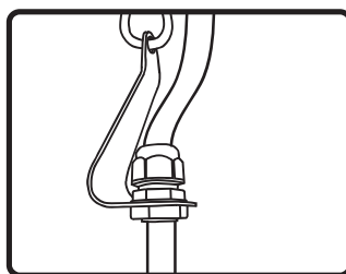
7. ケーブル吊り金具を使用する場合、取り付けブッシュを吊り金具に取り付け、信号線を通し高さを調整してブッシュを締め込みます。
