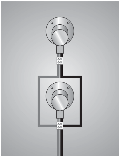
図3：高出力用の並列配線
