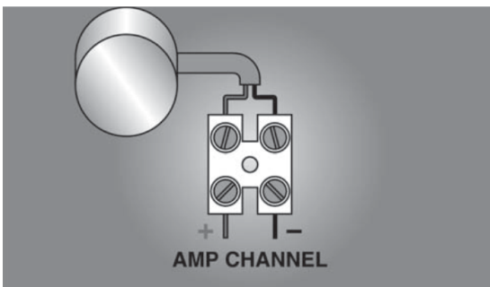
図2：ユーロスタイルコネクタ AMP CHANNEL：アンプのチャンネル
