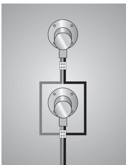
図3：高出力用の並列配線
