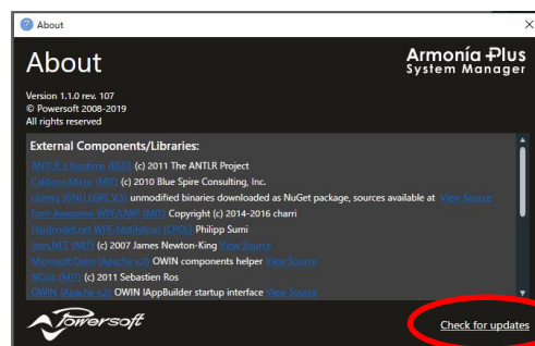
図 3 - About 画面
