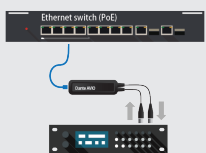
AES3対応パワーアンプへ
